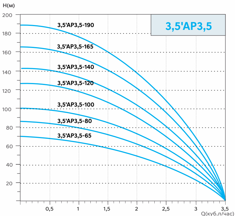
рисунок 1. График напорных характеристик
